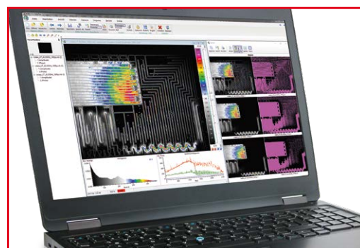
Analyse einer elektronischen Komponente durch Lock-In-Thermografie mit der Software IRIS® 3 active
